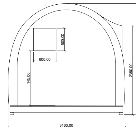
ELEWACJA WSCHODNIA
